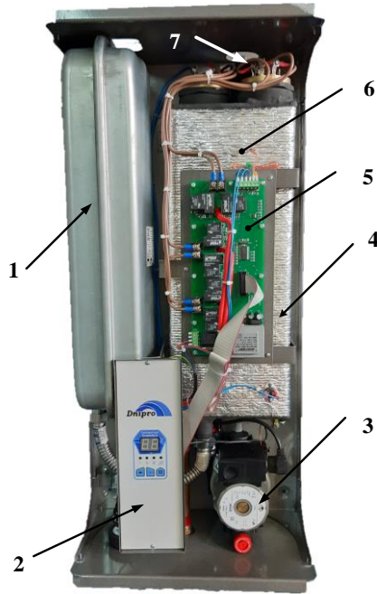
Рисунок 1 - Апарат електричний водогрійний КЕО-НС
